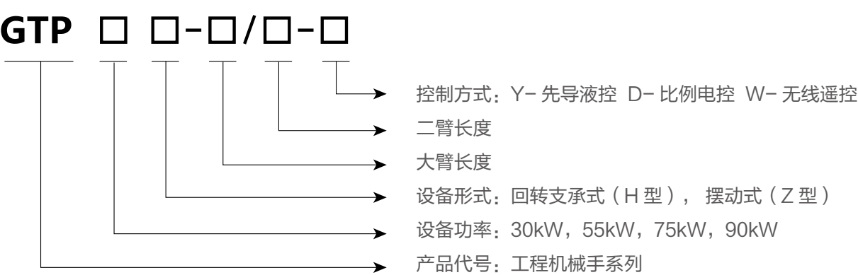
机械手主要参数 Machine Hand Parameters
